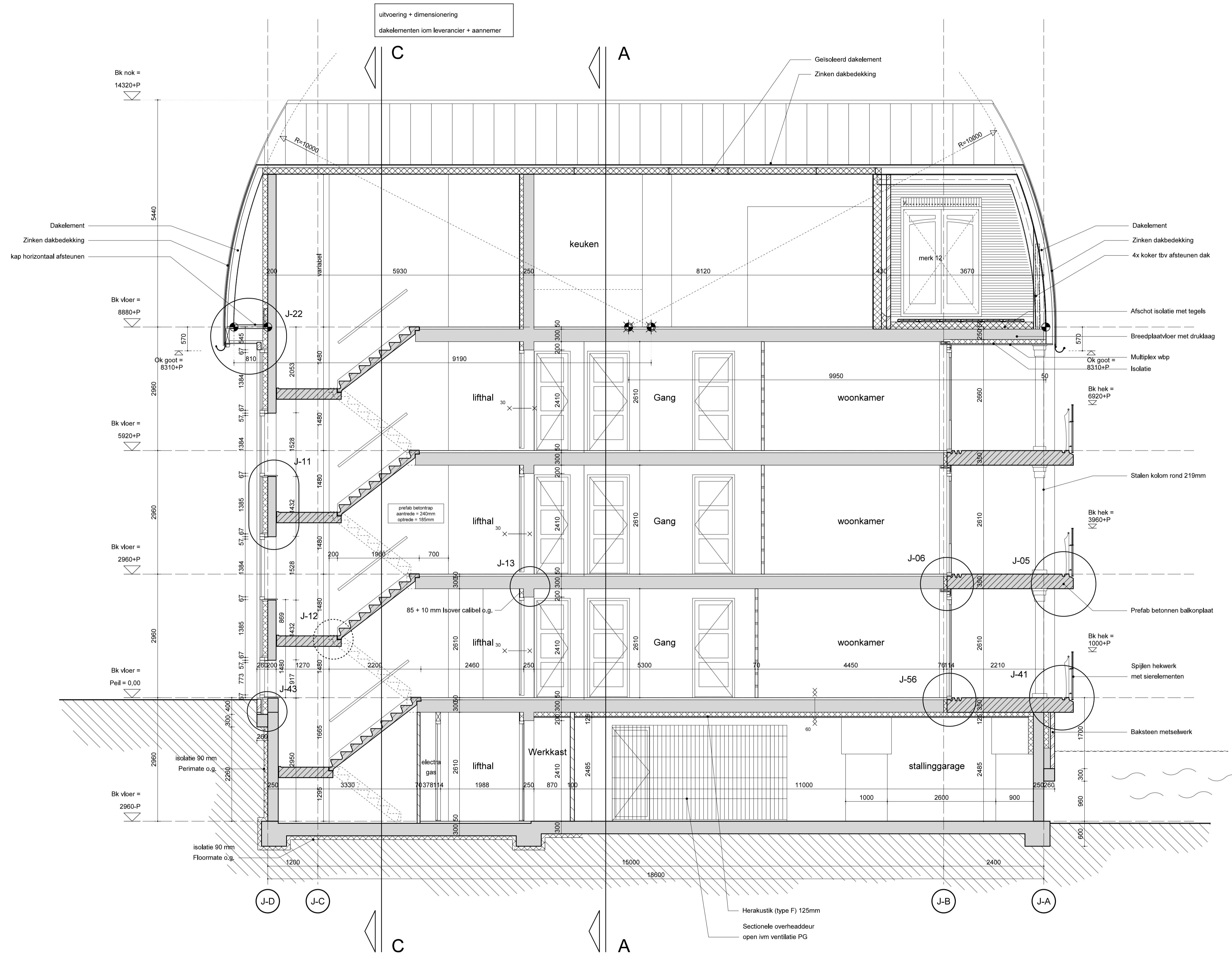
Doorsnede B-B
