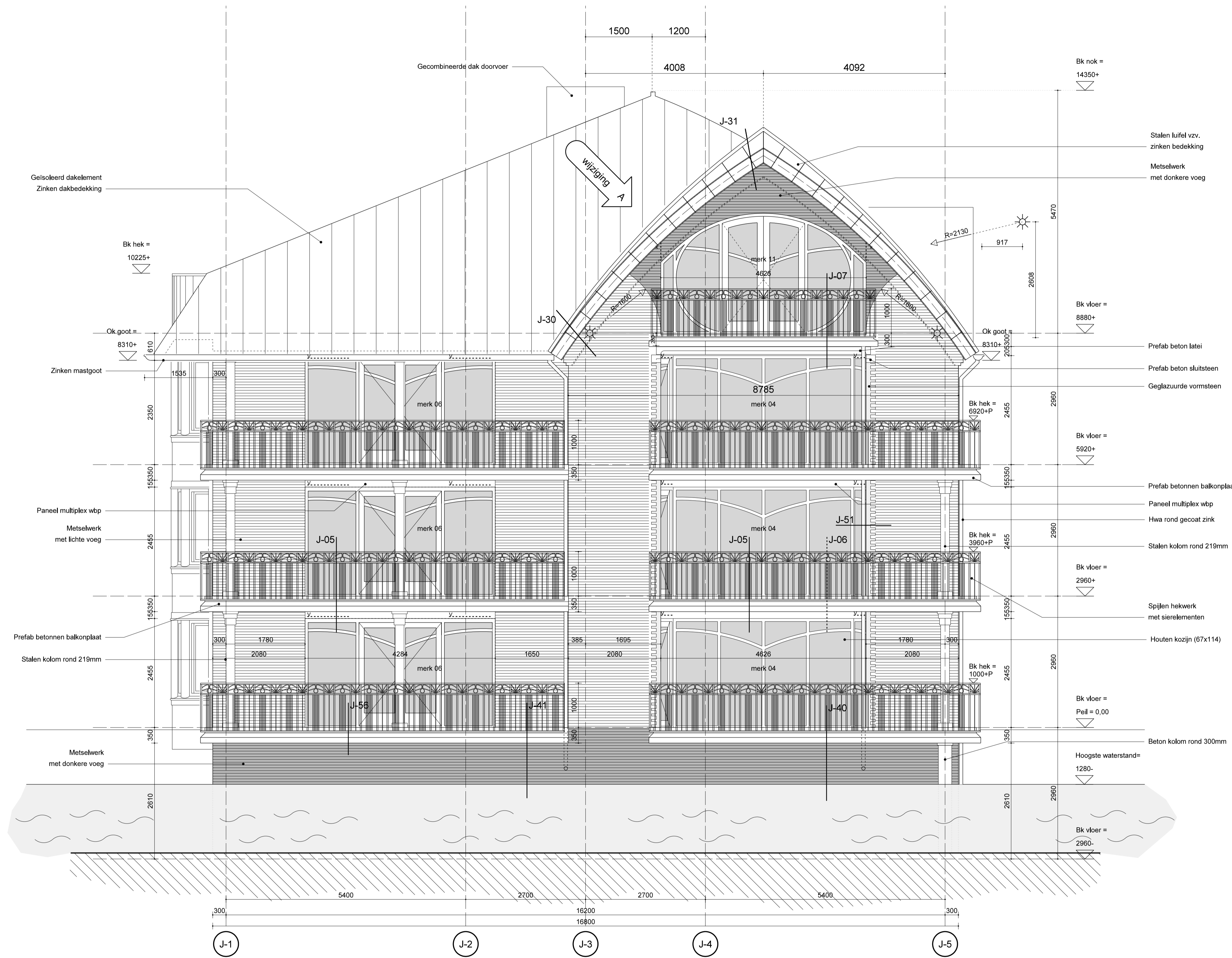
Zuid-oostgevel
